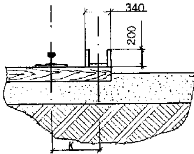
Рис. П.11.3. Лоток для укладки кабеля для кранов, оборудованный кабельным барабаном
