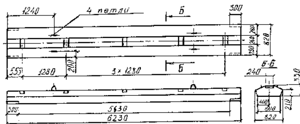
Рис. П.10.4. Железобетонная балка БРП-62.8.3
