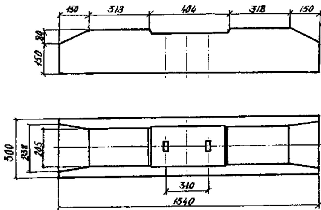
Рис. П.10.2. Железобетонная полушпала
