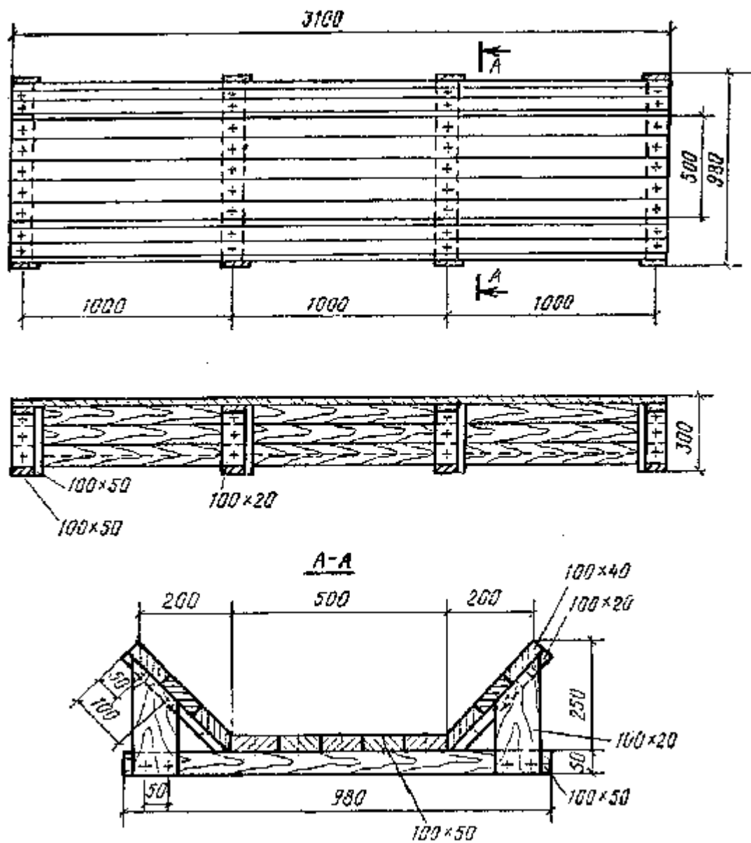
Рис. П.11.4. Лоток для укладки кабеля для кранов без кабельного барабана
