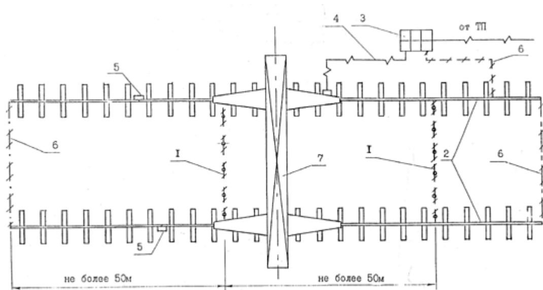
Рис. П.11.5. Схема заземления кранового пути
