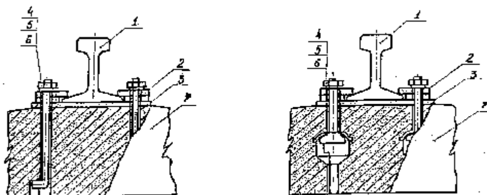
Рис. П.10.6. Прикрепление рельсов к железобетонным элементам разъемное:
