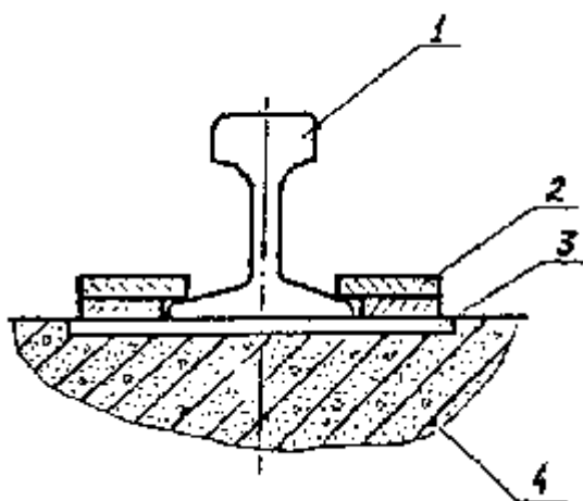
Рис. П.10.7. Прикрепление рельсов к железобетонным элементам неразъемное
