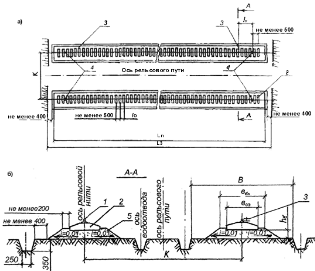
Рис. П.5.1. Рельсовый путь: а) - план; б) - поперечный профиль
