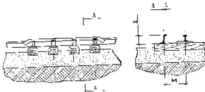
Рис. П.11.1. Ограничитель движения
