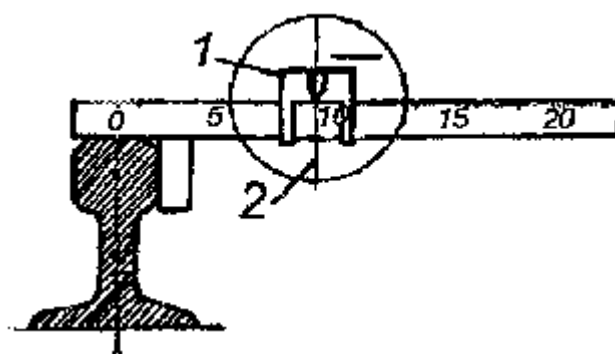
Рис. П.8.3. Переносная визирная линейка:
