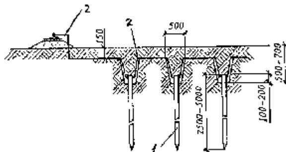
Рис. П.11.6. Схема соединения вертикальных заземлителей
