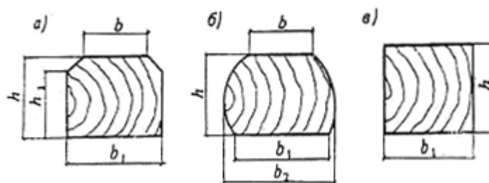
Рис. П.10.1. Поперечные сечения деревянных полушпал:
