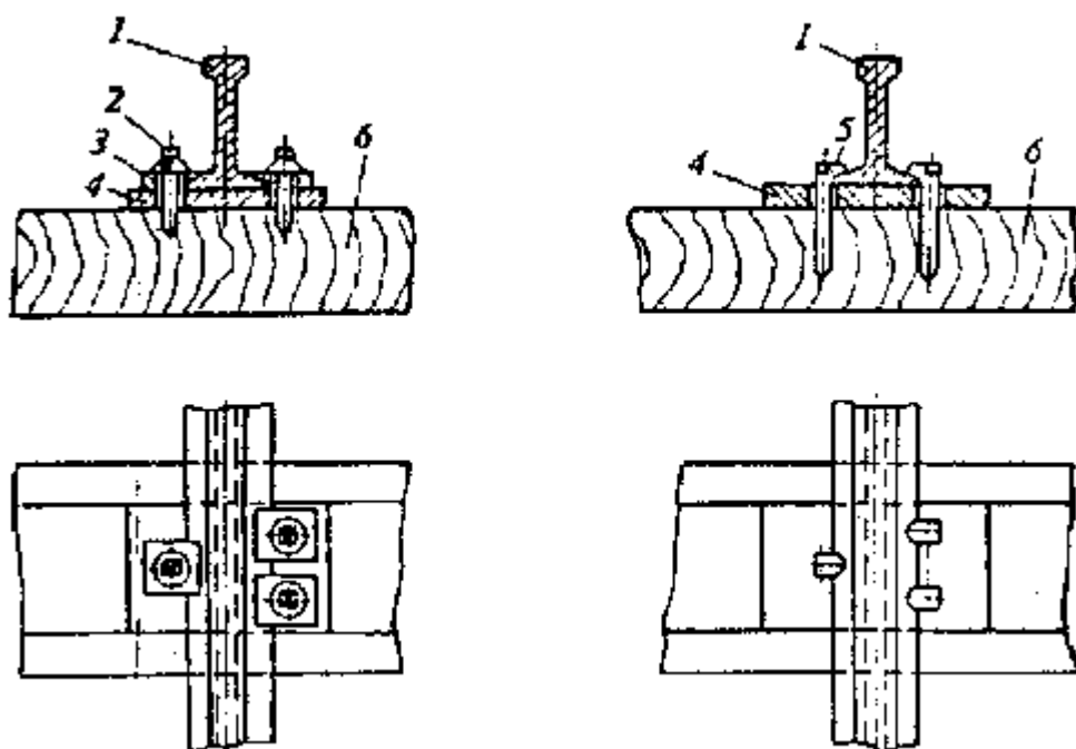
Рис. П.10.5. Прикрепление рельсов к полушпалам:
